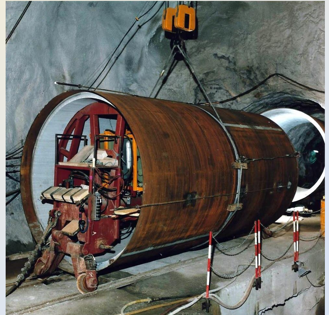
Oben: Verlegen der Rohre links: Montage der Stollenfräse für den Schrägschacht zum Krafthaus
